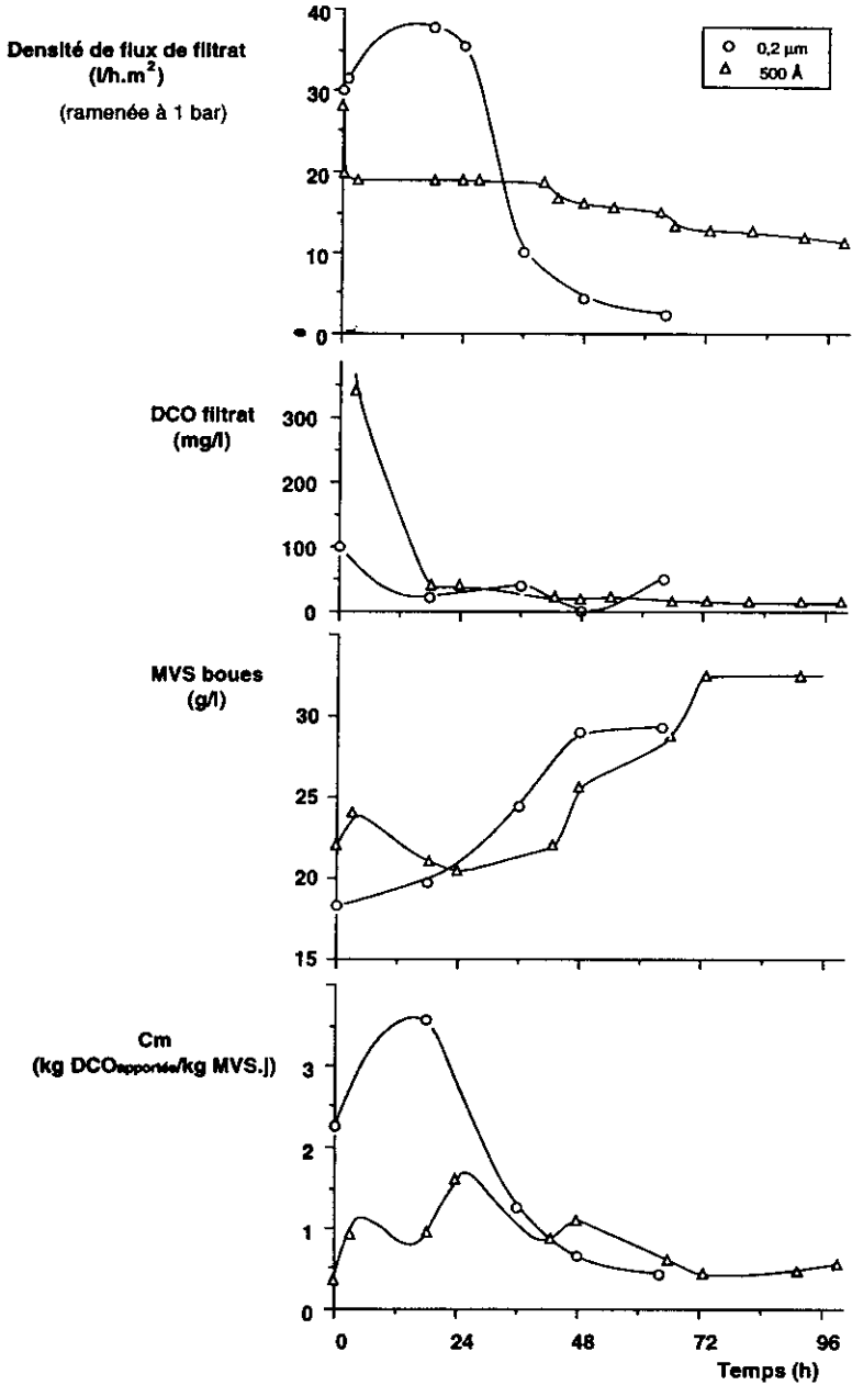
Figure 2 Suivi du flux de filtrat, de la DCO du filtrat, des MVS et de la charge mas- sique pour le traitement d'eau usée synthétique en recyclage total de biomasse sur membranes 0,2 µm et 500 Å.
