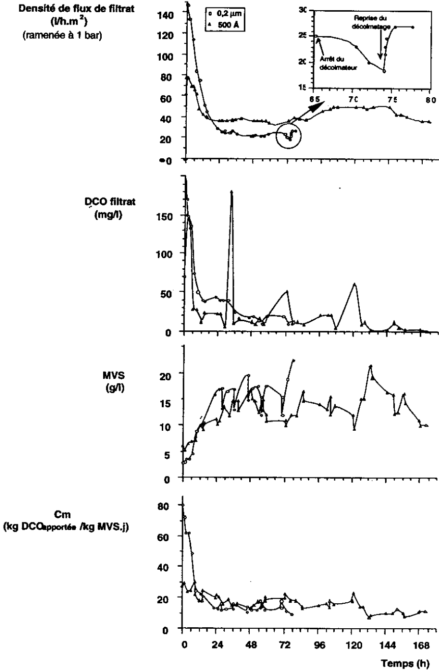
Figure 3 Suivi du flux de filtrat, de la DCO du filtrat, des MVS et de la charge massique pour le traitement d'eau usée synthétique sur membranes 0,2 µm et 500 Å.
