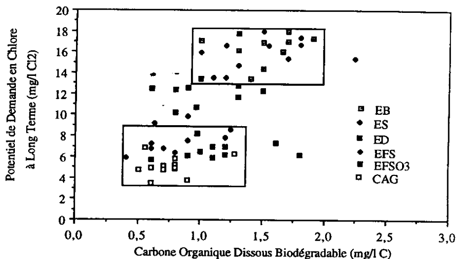
Figure 8 Tentatives de corrélation entre le potentiel de demande en chlore à long terme et le CODB pour l'ensemble des eaux de la filière.
